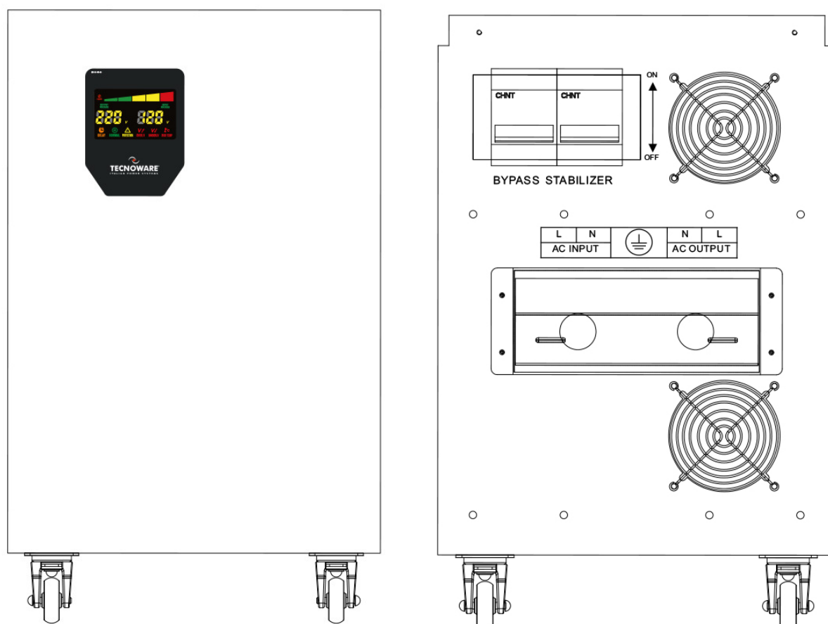
Figura 5 - Fronte e Retro (modelli FSTEL9M, FSTEL12M, FSTEL18M, FSTEL25M, FSTEL35M)
