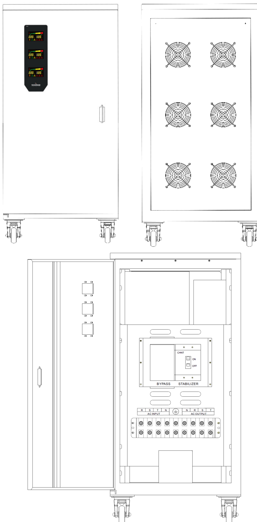
Figure 7 - UP: Front side, rear side - DOWN: Front side with open door (FSTEL50KT, FSTEL55KT, FSTEL60KT, FSTEL75KT, FSTEL100KT, FSTEL120KT models)
