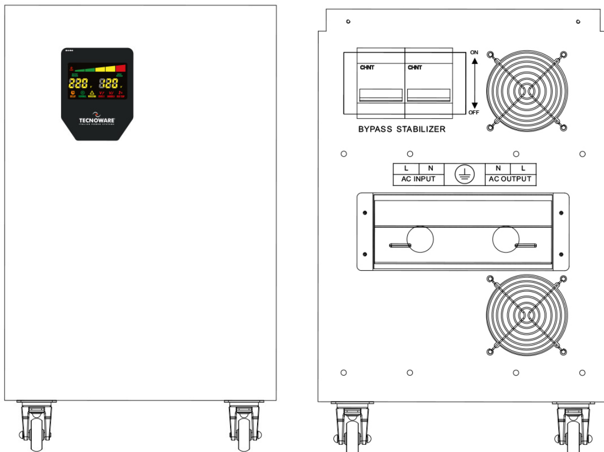
Figure 5 - Front side and rear side (FSTEL9KM, FSTEL12KM, FSTEL18KM, FSTEL25KM, FSTEL35KM models)
