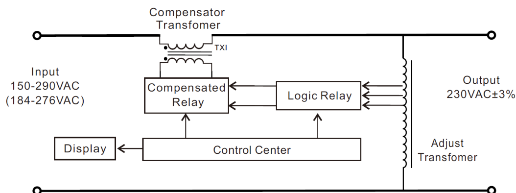
Figura 1 - Diagrammi a blocchi dello Stabilizzatore Elettronico
